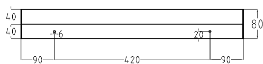
widok z tyłu rozmieszczenie otworów montażowych
