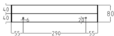
widok z tyłu rozmieszczenie otworów montażowych
