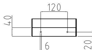
widok z tyłu rozmieszczenie otworów montażowych
